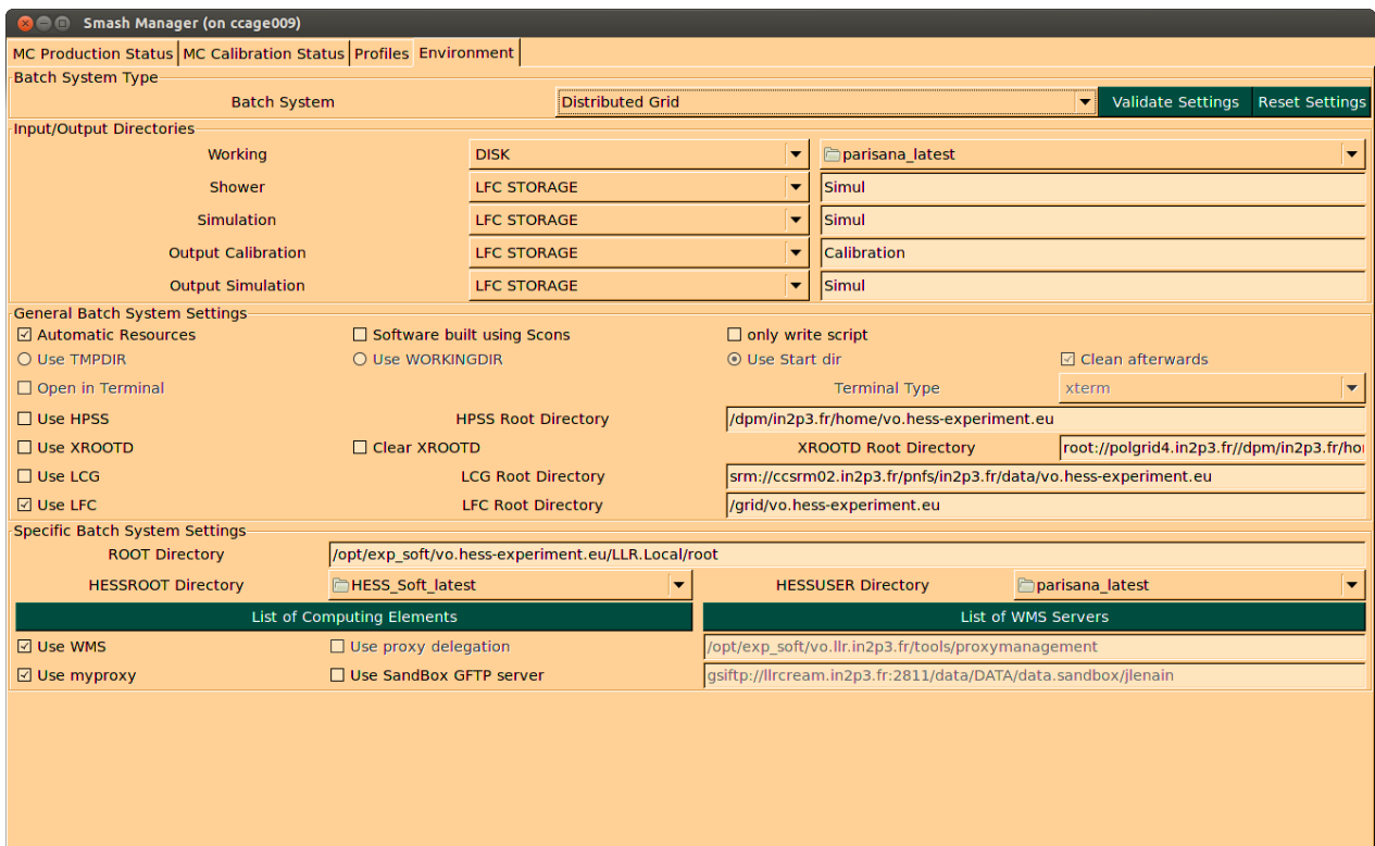
Figure 2: Exemple de l'interface graphique du logiciel d'analyse ParisAnalysis, montrant ici l'implémentation de l'environnement grille EGI pour la soumission de jobs. (Example of the ParisAnalysis analysis software graphical user interface, presenting here the implementation of the EGI grid environment for job submission.)
